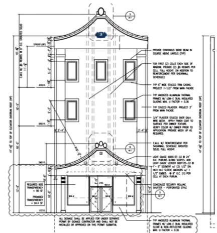
芝加哥服務中心設計藍圖。圖片來源 / 慈濟芝加哥分會
